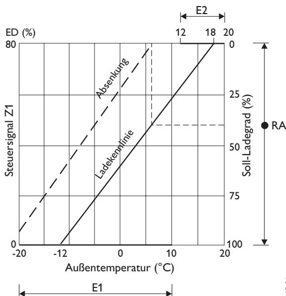
Absenkung der Aufladung durch Ansteuerung von Klemme KU
