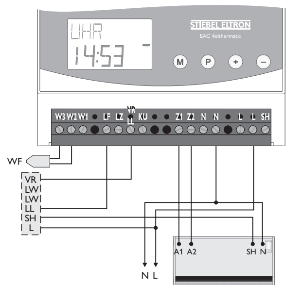
Anschlussschema Powertherm
